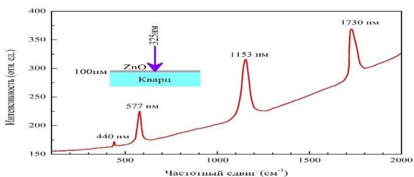
Рис.2. Спектр РРР, измеренный в плёнке ZnO. Длина волны возбуждения 325 нм
