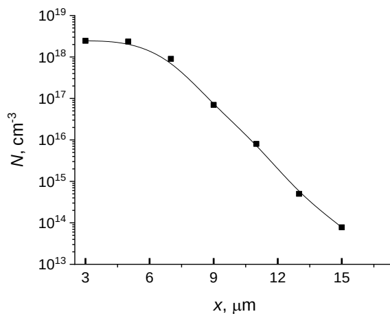
Рис. 3. Распределение концентрации атомов европия в кремнии после диффузии в интервале температур T=1250^\circ\text{C} в течение t=15 ч.
