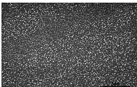
1-rasm. Ni yupqa qatlamini Ar gazi muhitida haroratning 100 °C, 300 °C va 500°C qiymatlarida qizdirilgandan keyin olingan SEM tasvirlari va shakllangan Ni nanozarrachalar gistogrammasi.
