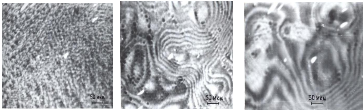
Рис.1. ИК-лазерная интрограмма n-Si, после ступенчатого отжига по циклу а) 600°C, б) 600°C + 1100°C, в) 600°C + 900°C + 1100°C.
