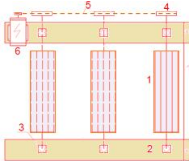
1-rasmda. Suvda suzuvchi girlyandli mikro gidroelektrostansiya.
