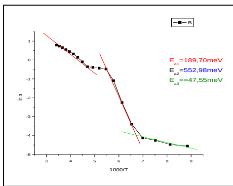
2-rasm: D4.2 namuna uchun o'tkazuvchanlikning temperaturaga bog'liqligi va aktivatsiya energiyalari
