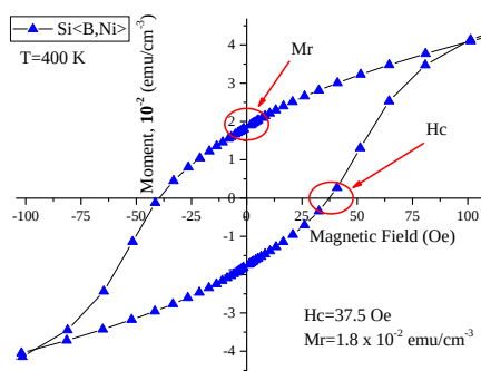
Рис. 2. Гистерезис петля в кремний легированного примесными атомами Ni при температуре T=400 \text{ K} .
