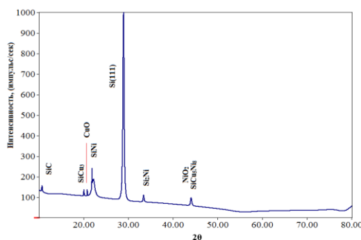
Рис.1. Рентгенограмма образца \text{n-Si<Ni,Cu>} до облучения
