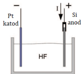
1-rasm. Anodik o'yish usuli orqali g'ovakli kremniy olish sxemasi [3]
