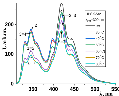
Рис. 2. Спектры ФЛ, возбужденные на длине волны 300 нм, исходного (1) и термообработанного при 30^\circ\text{C} (2), 40^\circ\text{C} (3), 50^\circ\text{C} (4), 60^\circ\text{C} (5), 70^\circ\text{C} (6) и 80^\circ\text{C} (7) образцов UPS-923A.
