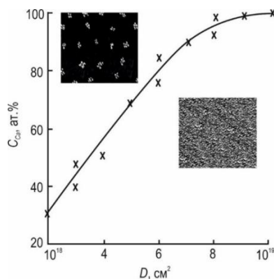
Рис. 1. Зависимость поверхностной концентрации Са от дозы облучения для \text{CaF}_2 , бомбардированного электронами с E_0 = 3 кэВ. На вставке РЭМ-изображения поверхности \text{CaF}_2 , бомбардированного электронами с E_e = 3 кэВ при D = 10^{18} \text{ см}^{-2} (а) и 10^{19} \text{ см}^{-2} (б).
