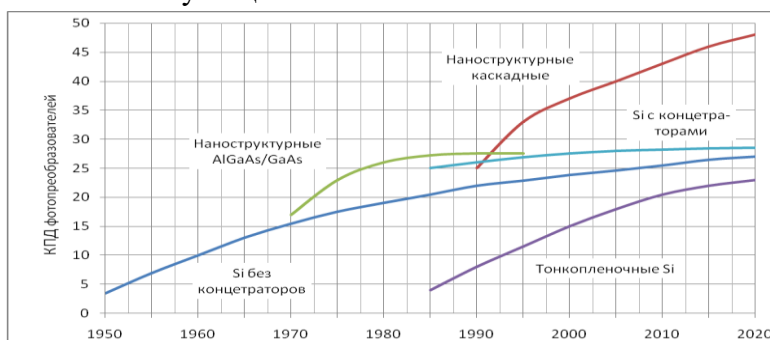
Рис. 2. Динамика увеличения КПД фотопреобразователей на основе кремния и наноструктур
