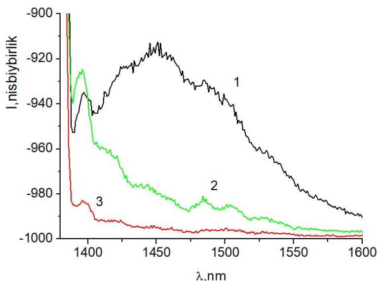
1-rasm. Surxon-18 \text{KMnO}_4 kaliy permanganat bilan legirlangan (1) va Yod ning 5% li spirtidagi eritmasi Surxon-18(2) hamda Yod ning 5% li spirtidagi eritmasi Surxon -104 paxta tolalarining fotolyumensensiya spektri.
