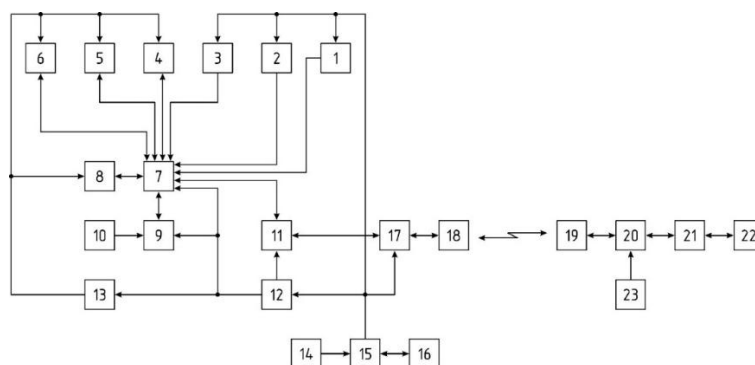
Рис. 1. Блок схема беспроводной метеостанции для непрерывного мониторинга метеопараметров окружающей среды
