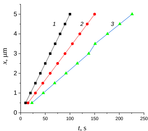
Рис. 1. Глубина травления от времени в образцах кремния легированного атомами европия при различных составах: 1 – 1\text{HF}+16\text{HNO}_3+8\text{CH}_3\text{COOH} , 2 – 1\text{HF}+16\text{HNO}_3+16\text{CH}_3\text{COOH} , 3 – 1\text{HF}+16\text{HNO}_3+24\text{CH}_3\text{COOH}
