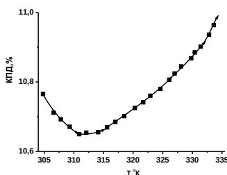
Рис.5. Температурная зависимость КПД CIGS ФЭМ
