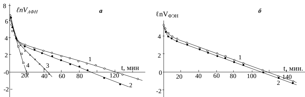
Рис. 1. Кривые релаксации V_{AФН} для АФН пленок CdTe:Ag (1, 2, 3), CdTe (4) (а) и кривые деполяризации «чистого» V_{ФЭН} для двух АФН пленок CdTe:Ag , полученных одновременно (б). E=293 К.
