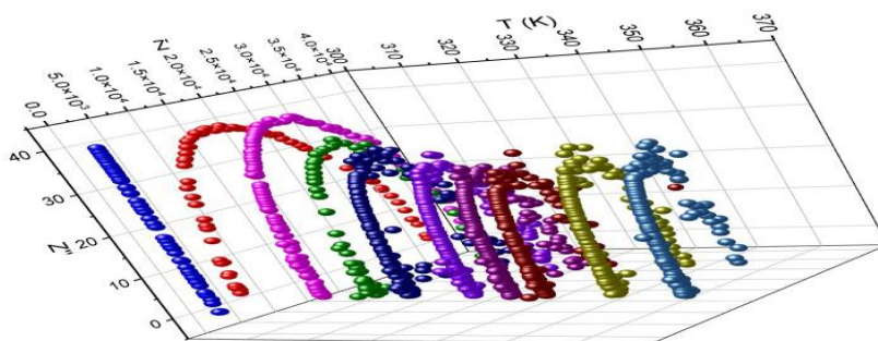
Рис. 2. Трёхмерная Найквист-диаграмма импеданса в координатах Z' - N - T для образца КДБ-3, где N — порядковый номер частотной точки
