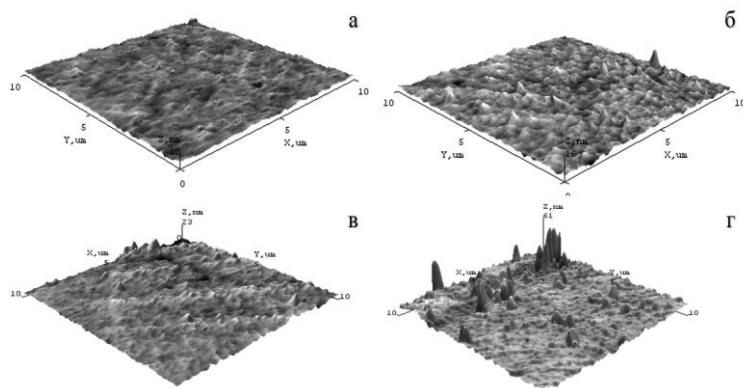
Рисунок 1. Трёхмерные АСМ-изображения поверхности плёнок CdS, осаждённых при 72 °С в течение различного времени: 5 (а), 10 (б), 15 (в), и 20 (г) минут
