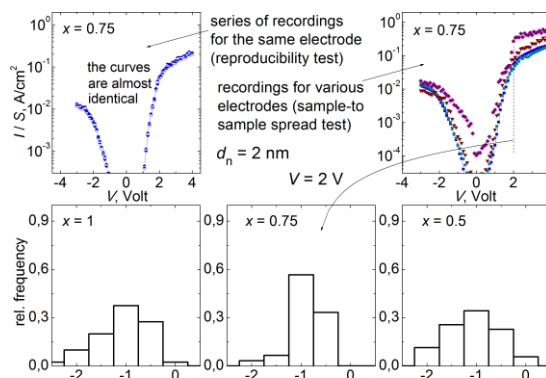
Рис. 2. Разброс характеристик
