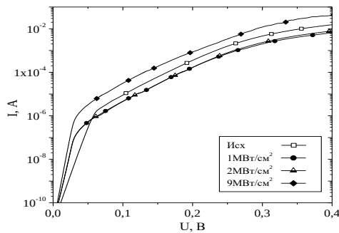
Рис.1. Зависимость прямого тока от напряжения при различных интенсивностях облучения ( T=300 \text{ K} ).
