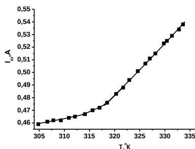
Рис.1. Температурная зависимость I_{K3} CIGS ФЭМ
