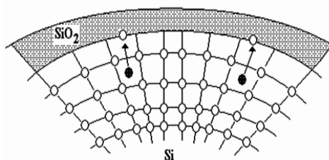
Рис. 2. Упрощенная модель уменьшения плотности поверхностных состояний за счет миграции примесных атомов в поле механических напряжений.
