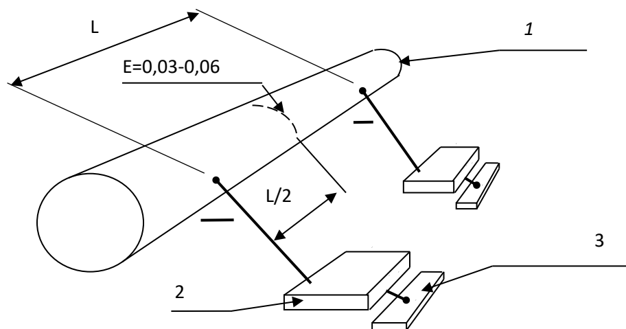
Рис.1. Схема присоединения источника электрического поля
