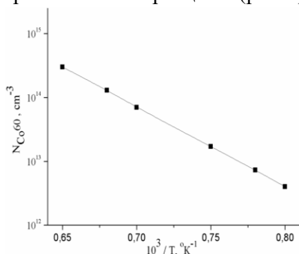
Рис. 1. Температурная зависимость электрически активная концентрация кобальта в n-Si
