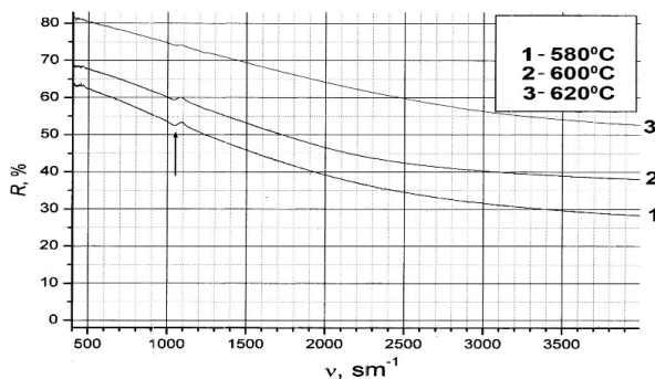
Рис 2 - Спектры отражения от образцов \text{TiSi}_2(\text{C49})/\text{Si} , обработанных при температурах 1 - 580°C, 2 - 600°C, 620°C
