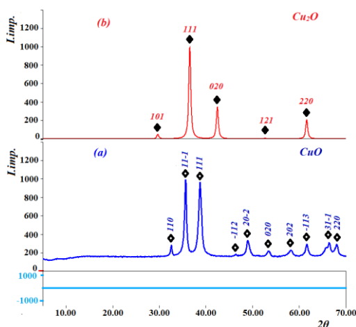
Рис. 1. Рентгенофазовый анализ пленок CuO и \text{Cu}_2\text{O} , выраженных на поверхности Si/ZnO.
