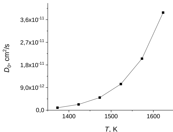
Рис. 2. Температурная зависимость коэффициента диффузии атомов европия в кремнии
