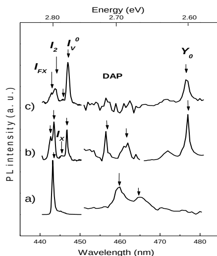
Рис.1 Типичные спектры ФЛ нелегированных образцов ЭС ZnSe/GaAs разной толщиной: 0.5 мкм (кривая а), 1.3 мкм (кривая б), 2 мкм (кривая в).
