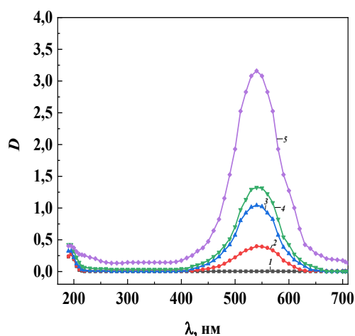
Рис 2. Спектры поглощения исходного (1) и облученного гамма лучами дозой 10^5 рад (2), 10^6 рад (3), 10^7 рад и 10^8 рад (5) кристаллов KCl
