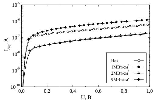
Рис.2. Зависимость обратного тока от напряжения при различных интенсивностях облучения ( T=300 \text{ K} ).
