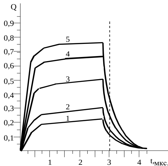
Рис.1. Зависимость коэффициента собирания носителей заряда
