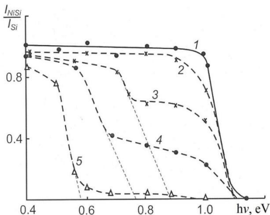
Рис.2. Зависимости интенсивности проходящего света от энергии фотонов для Si (111), имплантированного ионами \text{Ni}^+ с E_0=25 \text{ кэВ} , при дозах D, \text{ см}^{-2} : 1 - 0; 2 - 2 \cdot 10^{14} ; 3 - 2 \cdot 10^{15} ; 4 - 8 \cdot 10^{15} ; 5 - 8 \cdot 10^{16} . Во всех случаях после имплантации проводился прогрев до T=800-900 \text{ К} .
