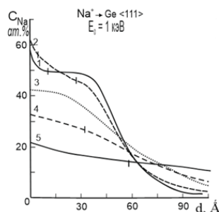
Рис. 2. Влияние отжига при различной температуре на распределение концентрации атомов натрия в германии, легированного ионами \text{Na}^+ с E_0 = 1 кэВ и D = 6 \cdot 10^{16} \text{ см}^{-2} . а) T , К: 1 – 300; 2 – 600; 3 – 900; 4 – 1100; 5 – 1300.
