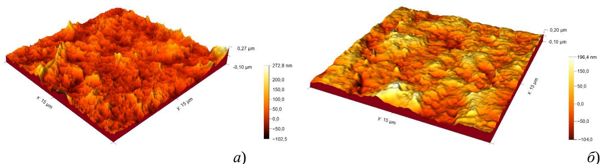
Рис.- 1. Морфология поверхности полиэтилена низкой плотности: а –исходный образец; б- образец облученный тормозным излучением с поглощенной дозой 400 кГр.
