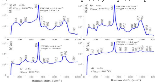
Рисунок 1. Спектры Рамана контрольных образцов n-Si и p-Si после термической обработки при температурах 1000°C и 1100°C.
