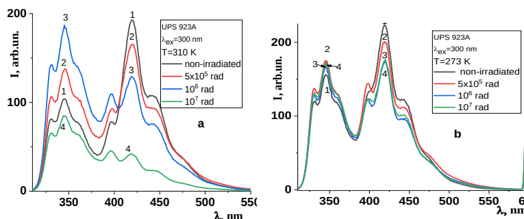
Рис. 1. Спектры ФЛ, возбужденные на полосе 300, исходного (1) и \gamma -облученного дозами 5 \times 10^5 Рад (2) 10^6 Рад (3) 10^7 Рад (4) образцов UPS - 923A, при температурах 310(а) и 273 (б)К.
