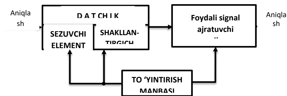
1-rasm. Sig'imli aniqlash datchigining umumiy shaklli sxemasi
