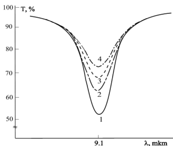
Рис.1. Типичные спектры ИК- поглощения контрольных образцов n- Si (кривая 1), n-Si<W> (кривая 2), n-Si+ВТО (кривая 3), n-Si<W>с предварительным ВТО при 1100^\circ\text{C} (кривая 4).
