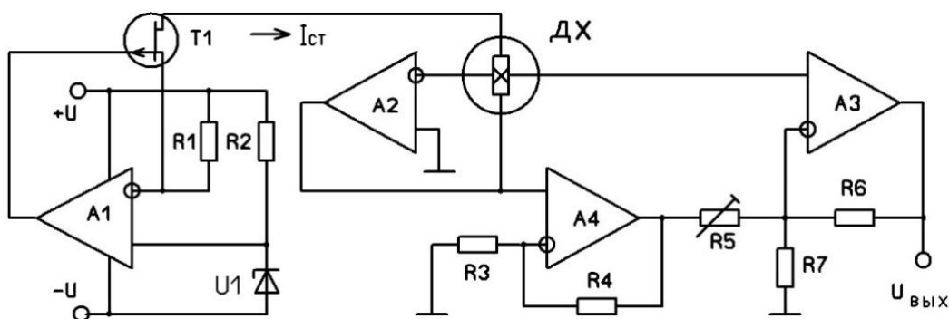
Рис.1. Структурная схема магнитометра.
