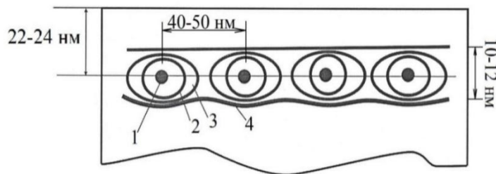
Рис. 1. Схематические изображения нанофаз (1-3) и нанослоя (4) \text{NiSi}_2 расположенных в приповерхностном слое Si. 1- D=2 \cdot 10^{14} \text{ см}^{-2} ; 2- 2 \cdot 10^{15} \text{ см}^{-2} ; 3- 8 \cdot 10^{15} \text{ см}^{-2} ; 4- 8 \cdot 10^{16} \text{ см}^{-2} .
