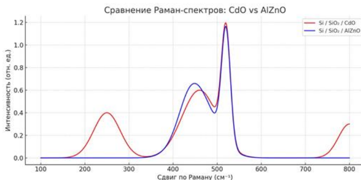
Рис.1. Раман-спектр структуры p-Si/SiO 2 -CdO и p-Si/SiO 2 - ZnAlO.
