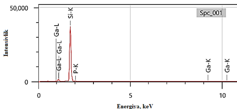
1-rasm. Kremniy sirtida hosil qilingan galliy fosfidi yupqa qatlamining element tarkibi
