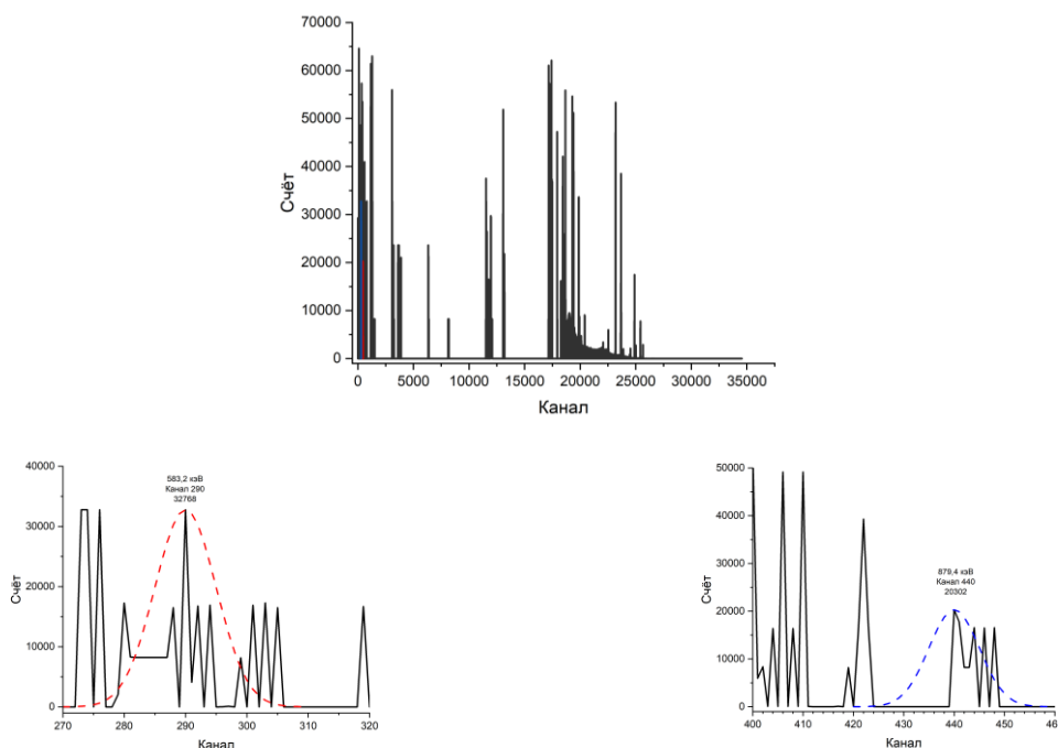
1-расм. n-Si<Tb> 1250^{\circ}\text{C} , 10 с., тез совутилган намунанинг гамма спектри
