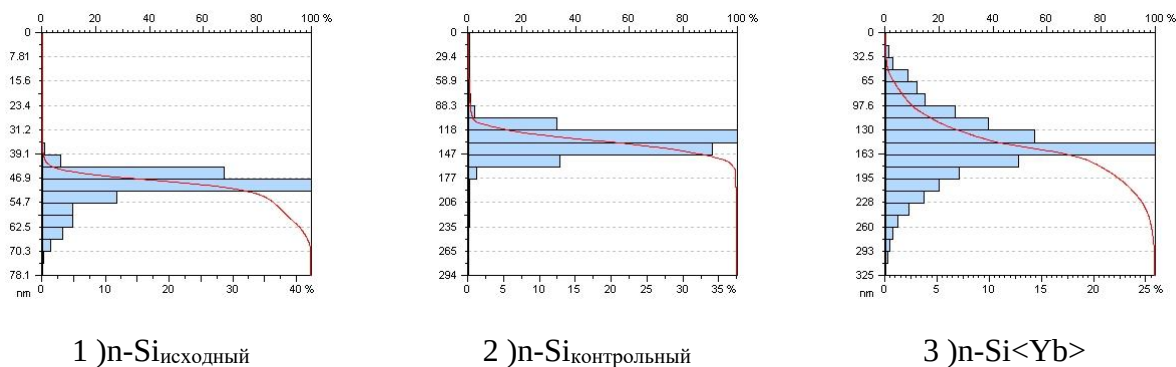
Рисунок 1. Изображения, полученные с помощью атомно-силовой микроскопии (АСМ): 1) Исходный образец n-Si; 2) Контрольный образец n-Si; 3) n-Si, легированный иттербием, со слоем 2 мкм, удаленным шлифованием после легирования
