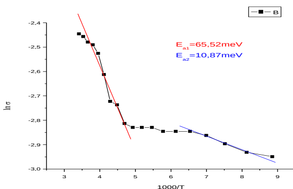
1-rasm: D3.3 namuna uchun o‘tkazuvchanlikning temperaturaga bog‘liqligi va aktivatsiya energiyalari
