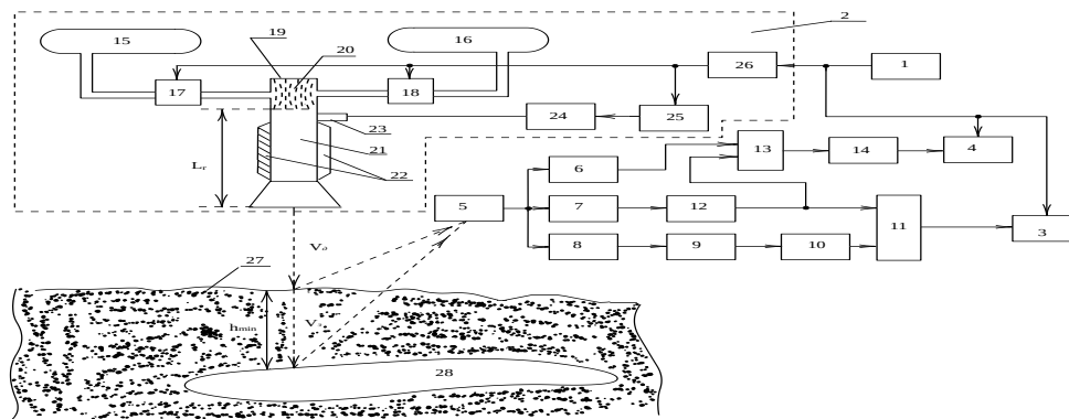
Рис. 1. Блок схема эхолокационного устройства
