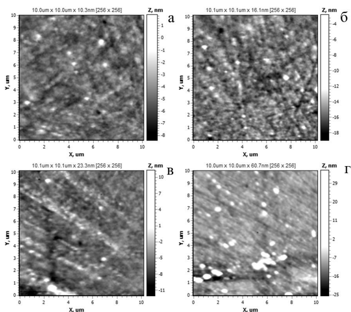
Рисунок 2. Двухмерные АСМ-изображения поверхности плёнок CdS, осаждённых при 72 °С в течение различного времени: 5 (а), 10 (б), 15 (в), и 20 (г) минут
