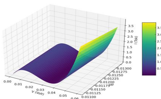
2-rasm. Yuqorida keltirilgan (7) ifodaga ko'ra ximpotensiallarning turli qiymatlarida tunnel tokining kuchlanishga bo'liqligi uch o'lchamdagi ko'rinishi
