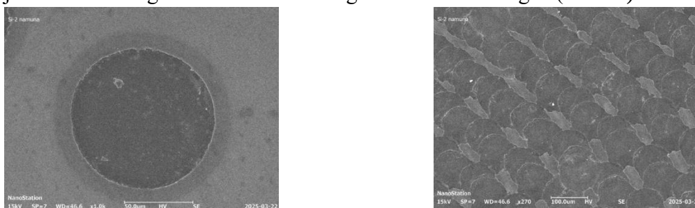
1-rasm. Kremniy sirtini morfologik tasvirlari. a) bitta impulsda b) 50 mm/min skanerlash tezligida
