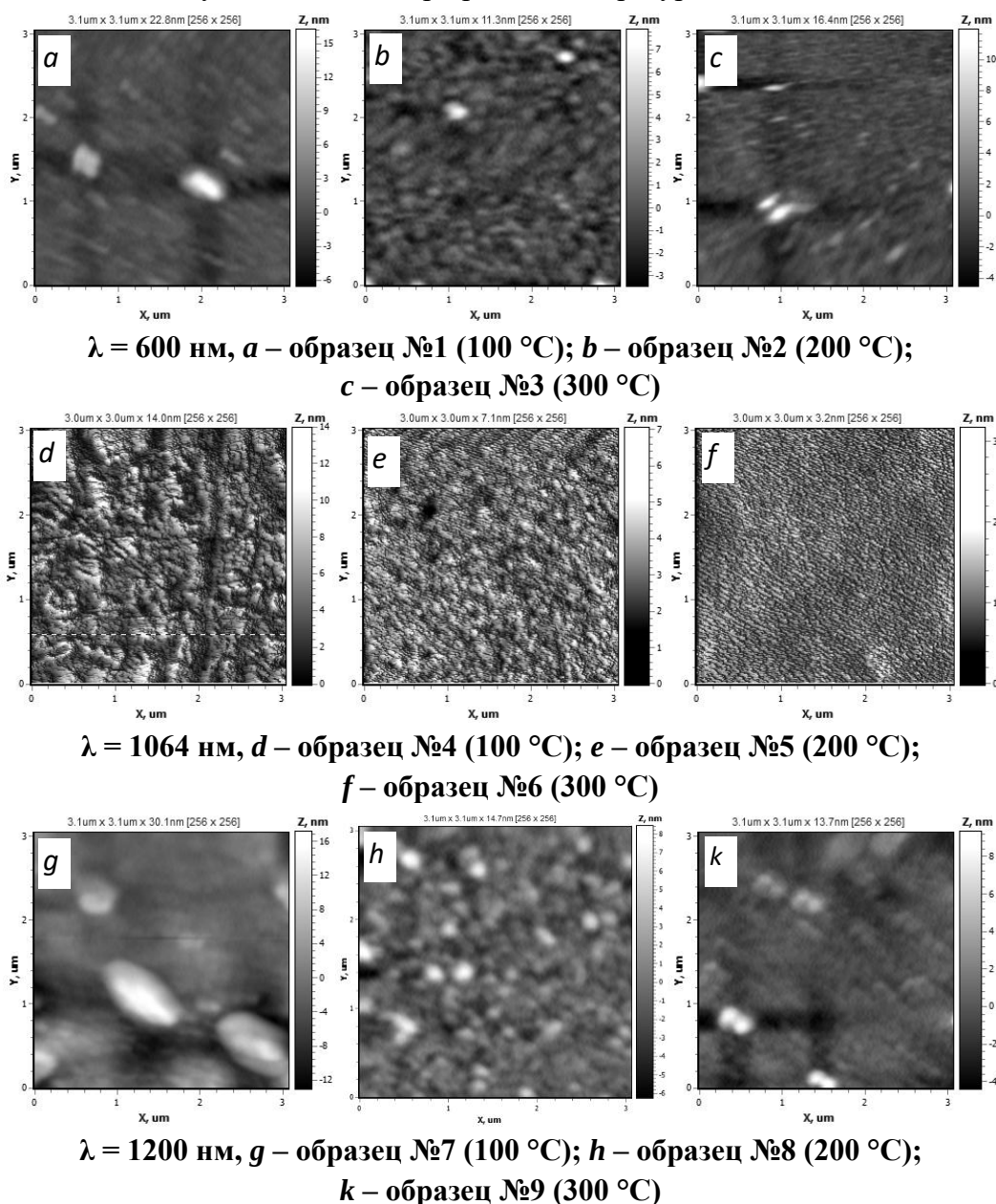
Рис.1. АСМ-изображения поверхности пленок CdTe, полученных при длине волны лазера 600 – 1200 нм и температуре подложки 100–300 °С
