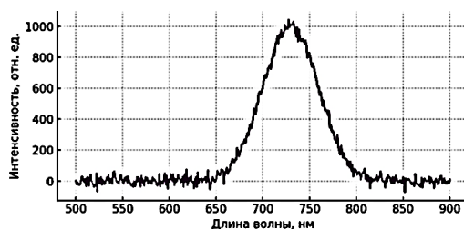
Рис.3. Фотолюминесцентные спектры после отжига до 1000°C.
