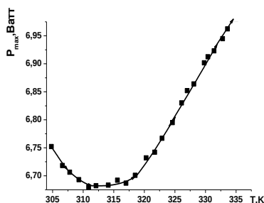
Рис.3. Температурная зависимость P_{max} CIGS ФЭМ
