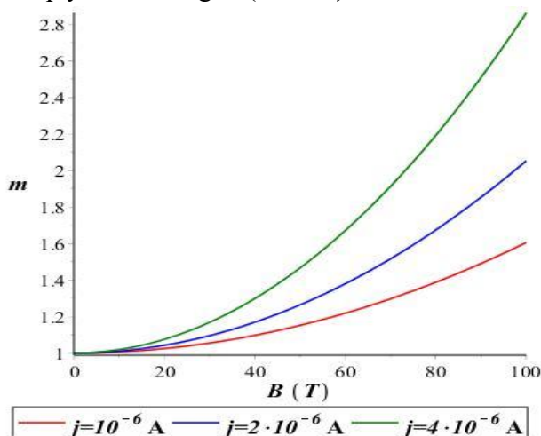
1-rasm. Noideallik koeffitsentini magnit maydon induksiyasi bog'lanishi
