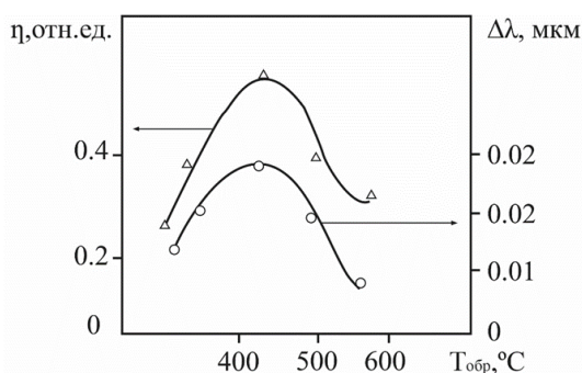
Рис.2. Изменение дифракционной эффективности ( \eta ) и сдвига края оптического поглощения ( \Delta\lambda ) пленок As_{40}Se_{60} , полученных из объёмных материалов с различной предысторией
