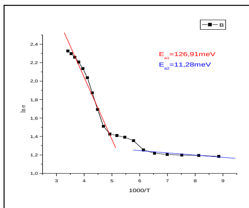
3-rasm: D4.4 namuna uchun o'tkazuvchanlikning temperaturaga bog'liqligi va aktivatsiya energiyalari
