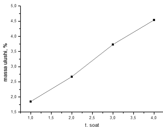
3-rasm. O'yish vaqti parametrining g'ovakli kremniy xossalariga ta'siri
