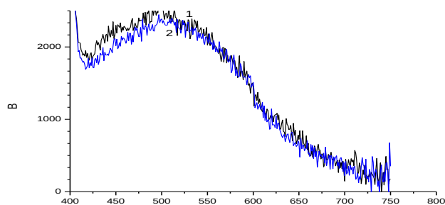
Рис 3- Спектры люминесценции TiSi 2 (C49) на кремнии 1 - 580°C, 2 - 620°C при возбуждении излучением спектрального состава полосы с максимумом ~375 нм и полушириной ~ 20 нм.
