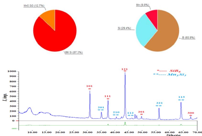
Рис. 1. Рентгенограмма образца КДБ-3: идентификация фаз \text{SiB}_6 (87,3 %) и \text{Mn}_5\text{Si}_3 (12,7 %).
