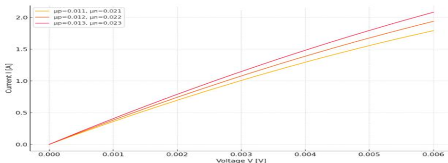
1-rasm. Yuqorida keltirilgan (7) ifodaga ko'ra ximpotensiallarning turli qiymatlarida tunnel tokining kuchlanishga bo'liqligi
