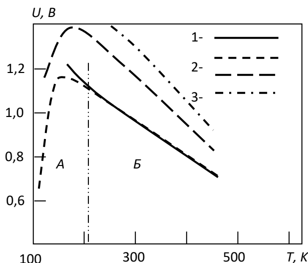
1-расм. Қуёш элементларининг салт ишлаш кучланишини температурага боғланиши. 1 - тажрибадан олинган натижалар [1], (9) формуладан олинган ҳисоблаш натижалари: 2- n=1 ; 3- n=1,1 ; ва 4- n=1,2 .
