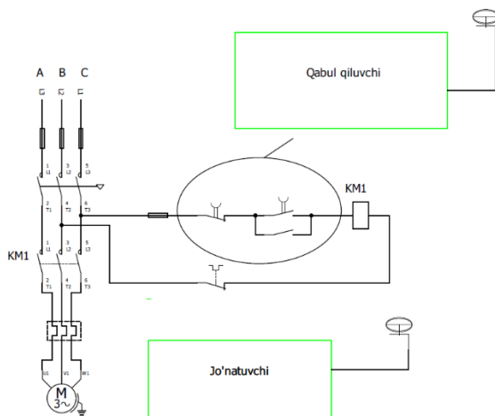
1-rasm. Elektr dvigatellarini radio aloqa bilan boshqaruv tizimi.
