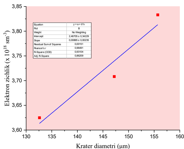
3-rasm. Al I (309,2 nm) FWHM yordamida aniqlangan plazma sohasidagi elektronlar zichligi krater diametri bilan chiziqli korrelyatsiyani ko'rsatadi
