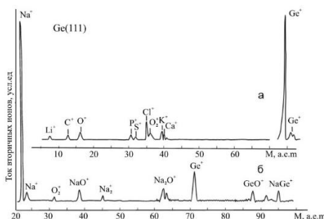
Рис. 1. Масс-спектры вторичных ионов чистого (а) и легированного ионами \text{Na}^+ с E_0 = 1 кэВ при D = 8 \cdot 10^{16} \text{ см}^{-2} (б) германия.
