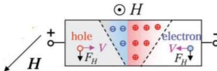
2 rasm. Magnit maydon ta'sirida p-n o'tishning hajmiy soha kengligini o'zgarishi [4; 2918-2923-b.]
