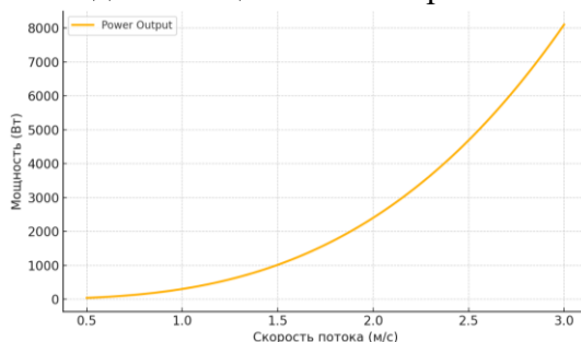
Рис.2. Зависимость выходной мощности от скорости потока воды
