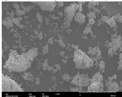
Рисунок 1. СЭМ-изображение порошка СаТiО 3
