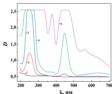
Рис.1. Спектры поглощения необлученного (1) и облученного \gamma -излучением дозами 10^5 Р (2), 10^6 Р (3), 10^7 Р (4) и 10^8 Р (5) кристаллов LiF
