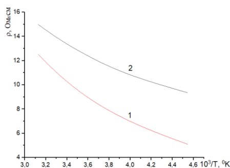
Рис. 2. Зависимость удельного сопротивления от температуры : 1– n- Si; 2– Ta/n-Si
