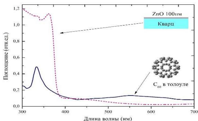
Рис. 1. Оптические спектры поглощения молекул фуллерена в растворе толуола (сплошная линия) и плёнки ZnO толщиной 100 нм (штриховая линия)
