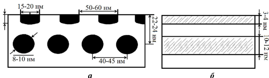
Рис. 3. Схематический разрез нанофаз (а) и нанослоев (б) \text{NiSi}_2 расположенных на поверхности и в приповерхностном слое \text{Si}(111)
