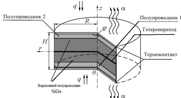
2-rasm. Variabentli yarimo'tkazgichning silindrik koordinatalardagi issiqlik fizikasi modeli.
