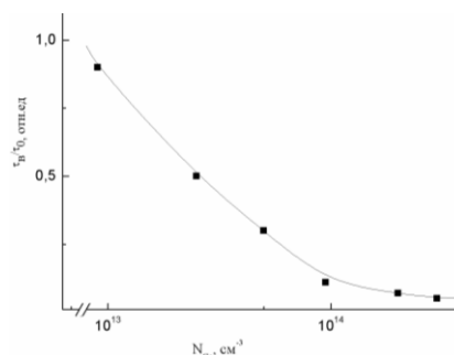
Рис. 2. Относительное изменение времени восстановления обратного сопротивление диодов из n-Si<Co> в зависимости от концентрации электрически активных рекомбинационных центров для образцов n-Si с \rho \approx 4 \Omega \cdot \text{см}
