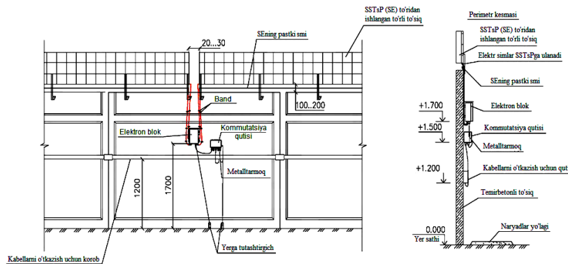
1.3-rasm. Sig'imli aniqlash datchigini devorda o'rnatish varianti
