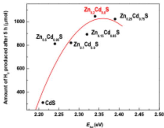
1-rasm. H_2 olinishining CdS va Zn_xCd_{1-x}S qattiq qotishmalarining taqiqlangan soha kengligiga bog'liqlik garfigi (5 soatlik reaksiyada olingan natija) [3]
