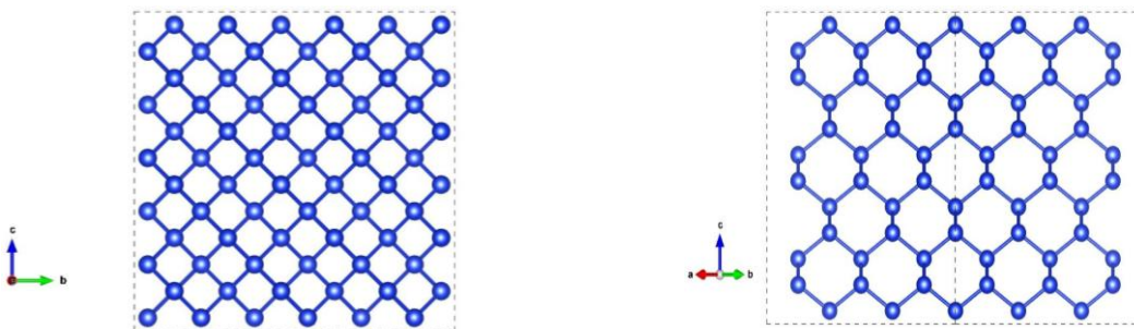
Рис. 1. Модель кристалла кремния, построенная в VESTA
