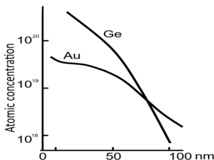
Рисунок 1. Профили распределения концентрации Ge и Au в GaAs
