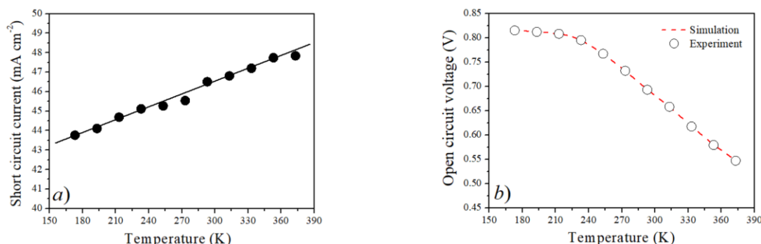
Рис. 1. Температурная зависимость тока короткого замыкания (a) и напряжения холостого хода (b) при 1367 Вт/м². Пунктирная линия – моделирование, окружность – эксперимент.
