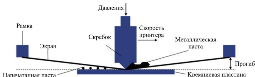
Рис. 1. Процесс трафаретной печати для металлизации солнечных элементов
