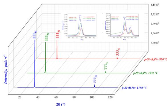
1-rasm. Pt atomlari diffuziyalangan p-Si<B,Pt> monokristall namunalarining 950°C, 1050°C va 1150°C haroratlarda 5 soat davomida otjog‘ qilinganidan keyingi rentgengrammlari.
