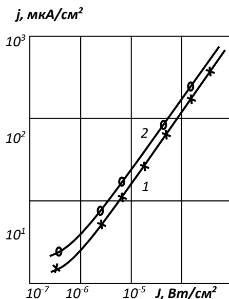
Рис. 1. Ватт-амперные характеристики газоразрядной ячейки при T=300 К и при разных значениях приложенного напряжения V . V равно: 1 – 1,5 кВ, 2 – 1,75 кВ.
