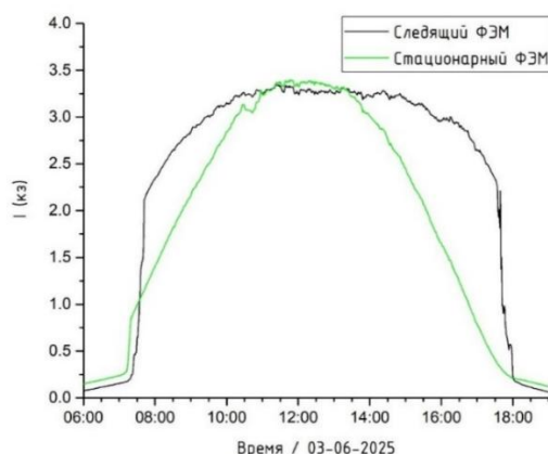
Рис. 1. График зависимости I_{кз} фотоэлектрических модулей от времени
