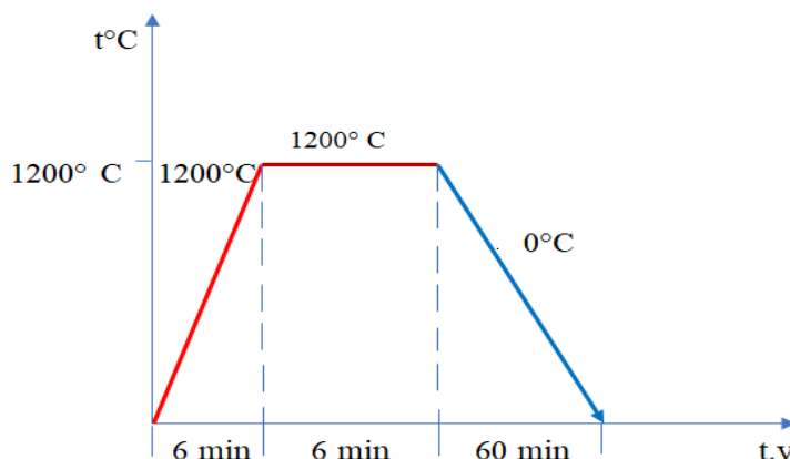
Рисунок 2. Температура формирования мишени из порошка \text{CaTiO}_3
