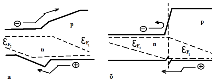
1-rasm. Geterobirlashmada zaryad tashuvchilarning injeksiyasi.
