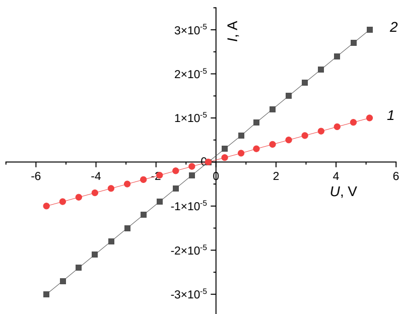
Рис. 1. Вольт-Амперная характеристика контакта кремния с Ga-In сплавом. 1 – обычный контакт, 2 – обработанный ультразвуком.
