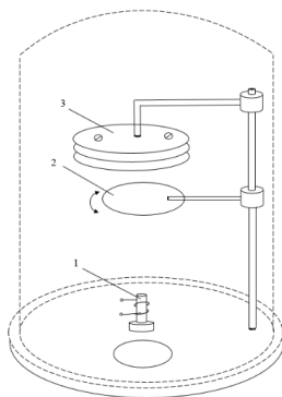
1-rasm. Vakuum kamerasining prinsipial sxemasi. 1-bug‘latgich, 2-ekran, 3-tutgichli taglik
