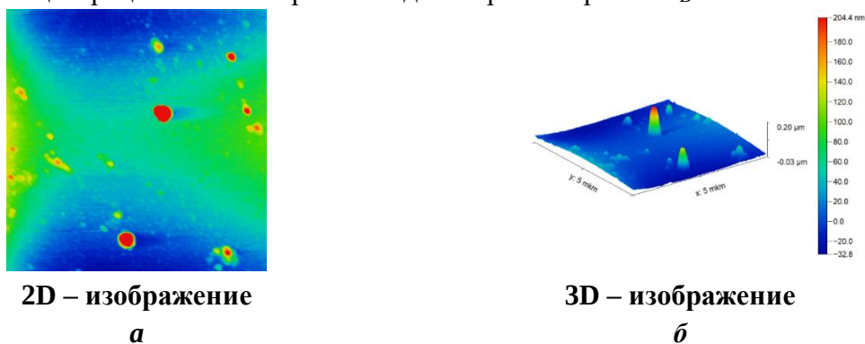
Рис. 1. Топография поверхности кремния после диффузии примесных атомов никеля, полученного в атомно-силовом микроскопе.
