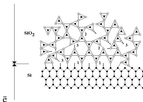
Рис. 1. Двумерная модель переходной области \text{Si-SiO}_2 . 1-оборванные валентные связи \text{Si} , 2- «мостиковый» кислород, 3- « не мостиковый» кислород.
