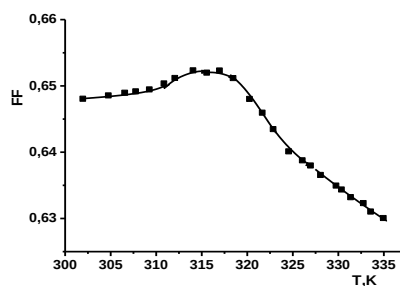
Рис.4. Температурная зависимость FF CIGS ФЭМ
