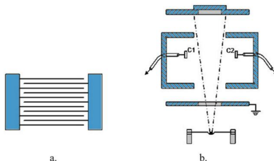
Рис. 1. Ёмкостной метод измерения толщины тонкого слоя:
