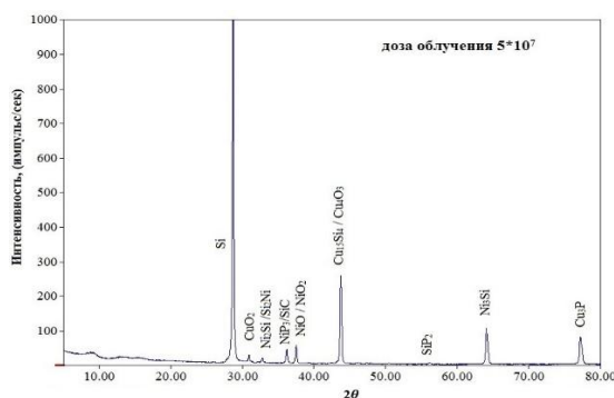
Рис.2. Рентгенограмма образца n\text{-Si}\langle\text{Ni,Cu}\rangle после \gamma -облучения дозой 5 \cdot 10^7 Рад
