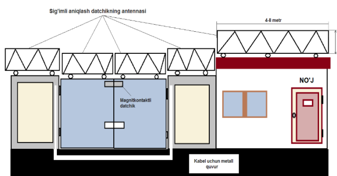
1.2-rasm. Datchikni darvoza va binolar ustida jihozlash chizmasi
