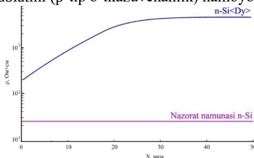
1-rasm. Disproziy atomlari bilan legirlangan n- va p-tipi kremniy namunalarining solishtirma qarshiligining chuqurlik bo'yicha taqsimoti ( T = 1200 \text{ } ^\circ\text{C} , t = 40 soat).
