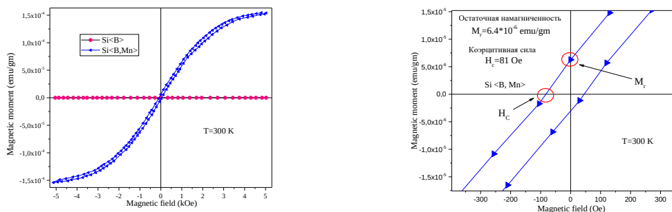
Рис. 1. Зависимость намагниченности от магнитного поля при T=300 \text{ K} , a - в образцах p -Si<B, Mn>, \rho=4 \cdot 10^4 \Omega \cdot \text{cm} (синий цвет) и исходного Si (красный цвет), b , нахождение параметров M_s , M_r , H_c .
