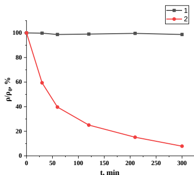
Рис. 1. Относительное изменение удельного сопротивления образцов кремния, легированном марганцем от времени отжига при T=100 °C: 1- с нанокластерами, 2- без нанокластеров.
