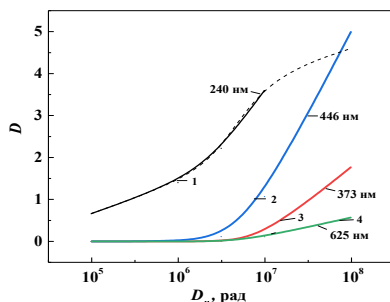
Рис.2. Дозовая зависимость изменения интенсивности поглощения F - (1), M - (2), R - (3) и N - центров (4) в гамма облученном кристалле LiF
