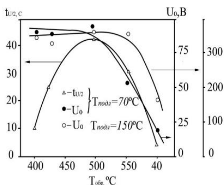
Рис.1 Зависимость предельного потенциала зарядки U_0 и времени полуспада потенциала в темноте ( t_{1/2} ) слоёв As_{40}Se_{60} от температуры обработки расплава исходного материала
