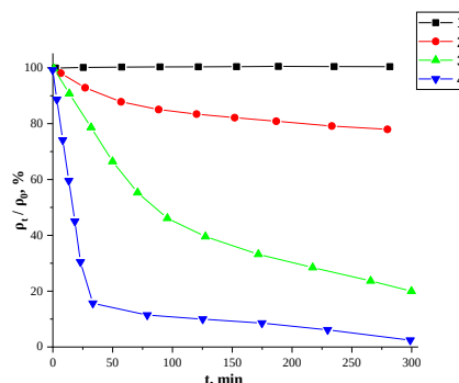
Рис. 2. Относительное изменение удельного сопротивления образцов кремния p -Si<B,Mn> с нанокластерами атомов марганца при различных температурах отжига: 1- 100 °C, 2- 125 °C, 3- 140 °C, 4- 160 °C.
