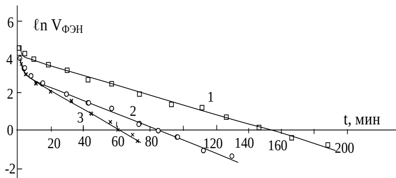
Рис. 2. Кривые деполяризации V_{ФЭН} для АФН пленок CdTe: Cd (кривая 1), CdTe: Cu (2) и Sb_2Se_3: Se (3) при T = 293 К.
