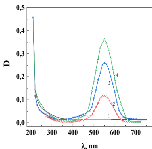
Рис 1. Спектры поглощения необлученного (1) и облученного рентгеновскими лучами дозой 12,564 рад (2), 41,88 рад (3) и 62,82 рад кристаллов KCl
