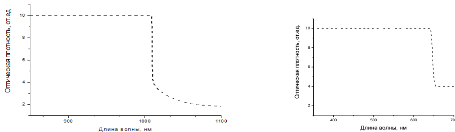
Рис. 1. Зависимость оптической плотности от длины волны: (а) для кремниевой подложки, (б) для силицида титана
