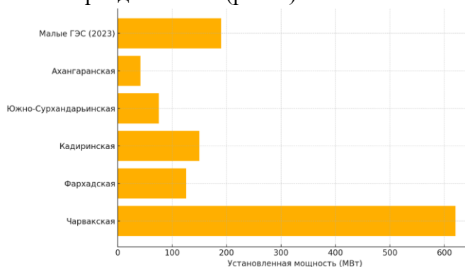
Рис.1. Установленная мощность крупнейших ГЭС Узбекистана [1]
