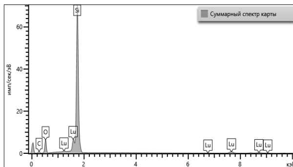
Рис.2. Концентрация элементов в кремнии, легированном лутецием
