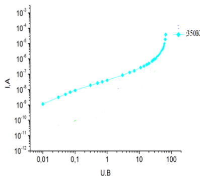
Рис. 1. Вольтамперная характеристика лавинного диода, легированного железом, при температуре 350К.
