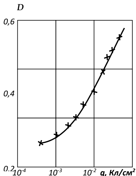
Рис. 2. Зависимость оптической плотности пленки висмута от «токовой» экспозиции q .
