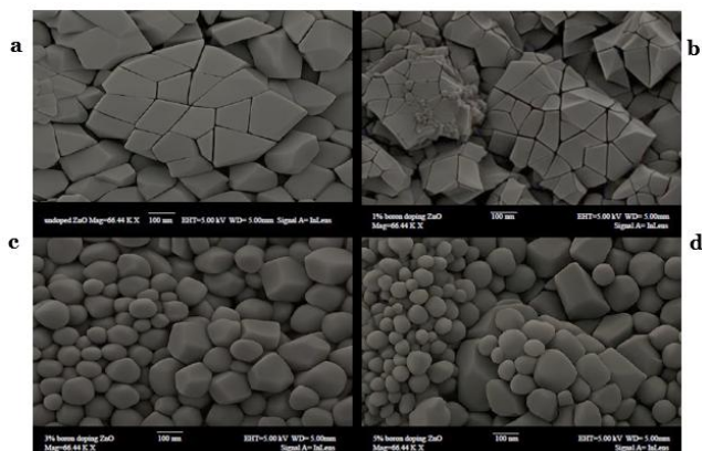
3-rasm. Sof va bor bilan legirlangan ZnO yupqa qatlamlarining SEM tasviri. a-sof ZnO, b-1%, c-3%, d-5%
