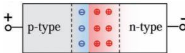
1 rasm. Magnit maydoni bo'lmaganda p-n o'tishning hajmiy zaryad soha kengligi [ 4; 2918-2923-b.]
