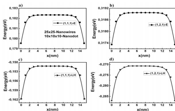
1-rasm. InAs nanonuqta (10×10×10 nm) InP/InAs 0.25 Po 0.75 /InP nanonaycha (25×25 nm) ichida har xil koordinatalarda joylashtirilganda elektron va yengil teshiklarning energiya darajalari qanday o'zgarishi ko'rsatilgan.
