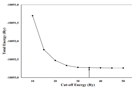
Рис. 2. Зависимость полной энергии кристалла кремния от энергии отсечения.
