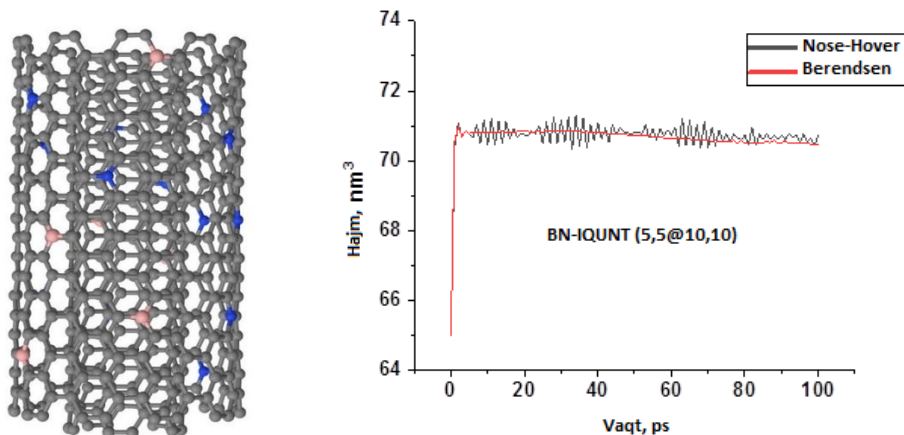
1-rasm. (5,5@10,10) xirallikdagi ikki qavatli uglerodli nanotrubka (chapda) va ushbu nanotrubkaning termo/barostatlarida qizdirilishi (o‘ngda).
