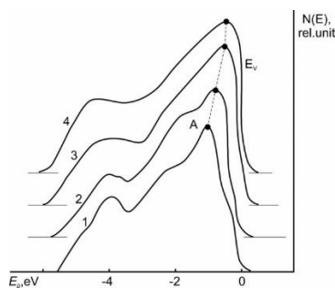
Рис. 1. КЭР фотоэлектронов для Si(111), бомбардированного ионами \text{Ar}^+ с E_0 = 1 кэВ при D , \text{cm}^{-2} : 1-0, 2- 2 \cdot 10^{14} , 3- 10^{15} , 4- 10^{16} .
