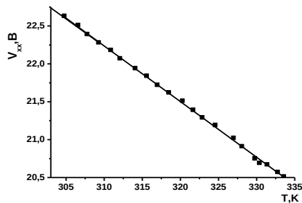
Рис.2. Температурная зависимость V_{xx} CIGS ФЭМ
