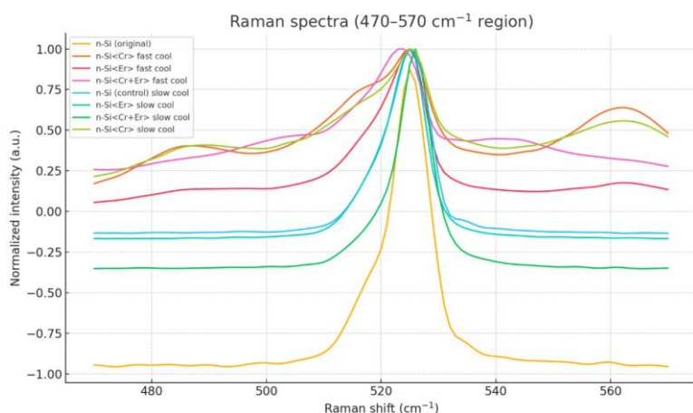
Рисунок 2. Фрагмент Раман-спектров в области 470–570 \text{см}^{-1} для образцов n-типа кремния: исходного (n-Si original), контрольного (n-Si control) и легированных Cr, Er и Cr+Er с последующим быстрым или медленным охлаждением.
