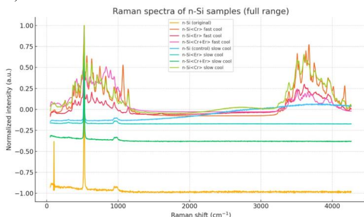
Рисунок 1. Полный спектральный диапазон нормализованных спектров комбинационного рассеяния (Рамана) для образцов n-типа кремния: исходный (n-Si original), контрольный (n-Si control) и легированные хромом (Cr), эрбием (Er) и их комбинацией (Cr+Er) при различных режимах охлаждения (быстрое и медленное охлаждение).
